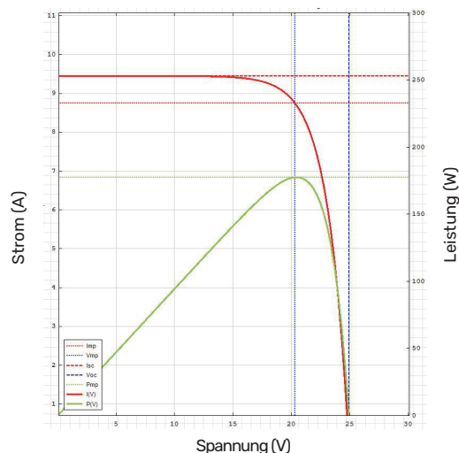
RNG-175DB-H Eigenschaften gegenüber der Spannung
